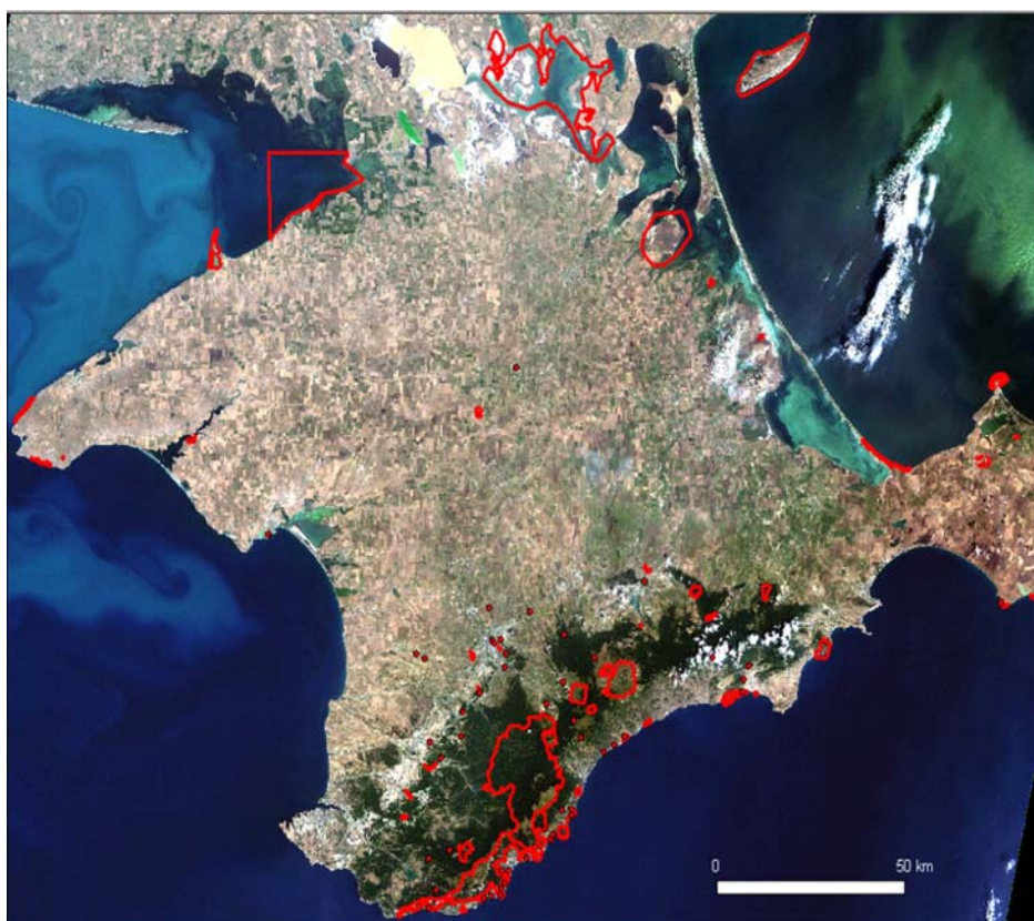
Рис. 1. Мозаїка території Криму на базі знімків “Landsat-7”
