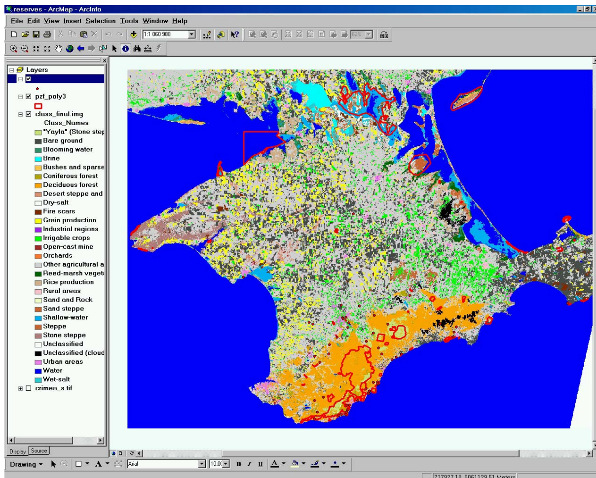
Рис. 2. Класифікація земної поверхні в ГІС УЦМЗР із контурами заповідних територій АР Крим
